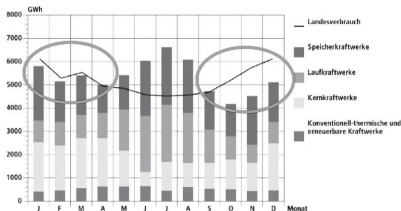
Monatliche Erzeugungsanteile und Landesverbrauch im Kalenderjahr 2021
