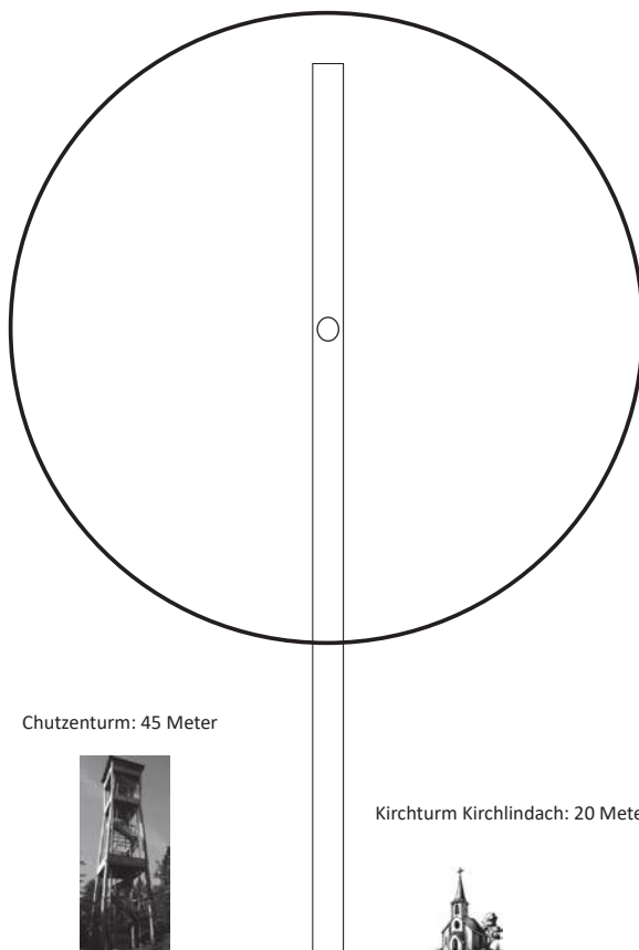
Höhe Windrad: 200 Meter, Rotordurchmesser: 140 Meter, Nabenhöhe: 140 Meter
